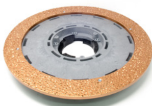
Tytan Ring \varnothing 430\text{mm} Per rimuovere colle cementizie vecchie, resine, graffiare pavimenti e asportare cordonature e sovra-spessori
